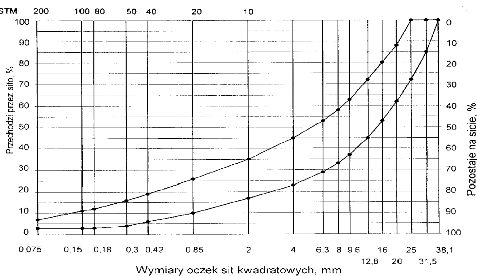
Rys.1. Krzywe graniczne uziarnienia mieszanki mineralnej BA od 0 do 31,5 mm do podbudowy nawierzchni drogi o obciążeniu ruchem KR 1 lub KR 2
