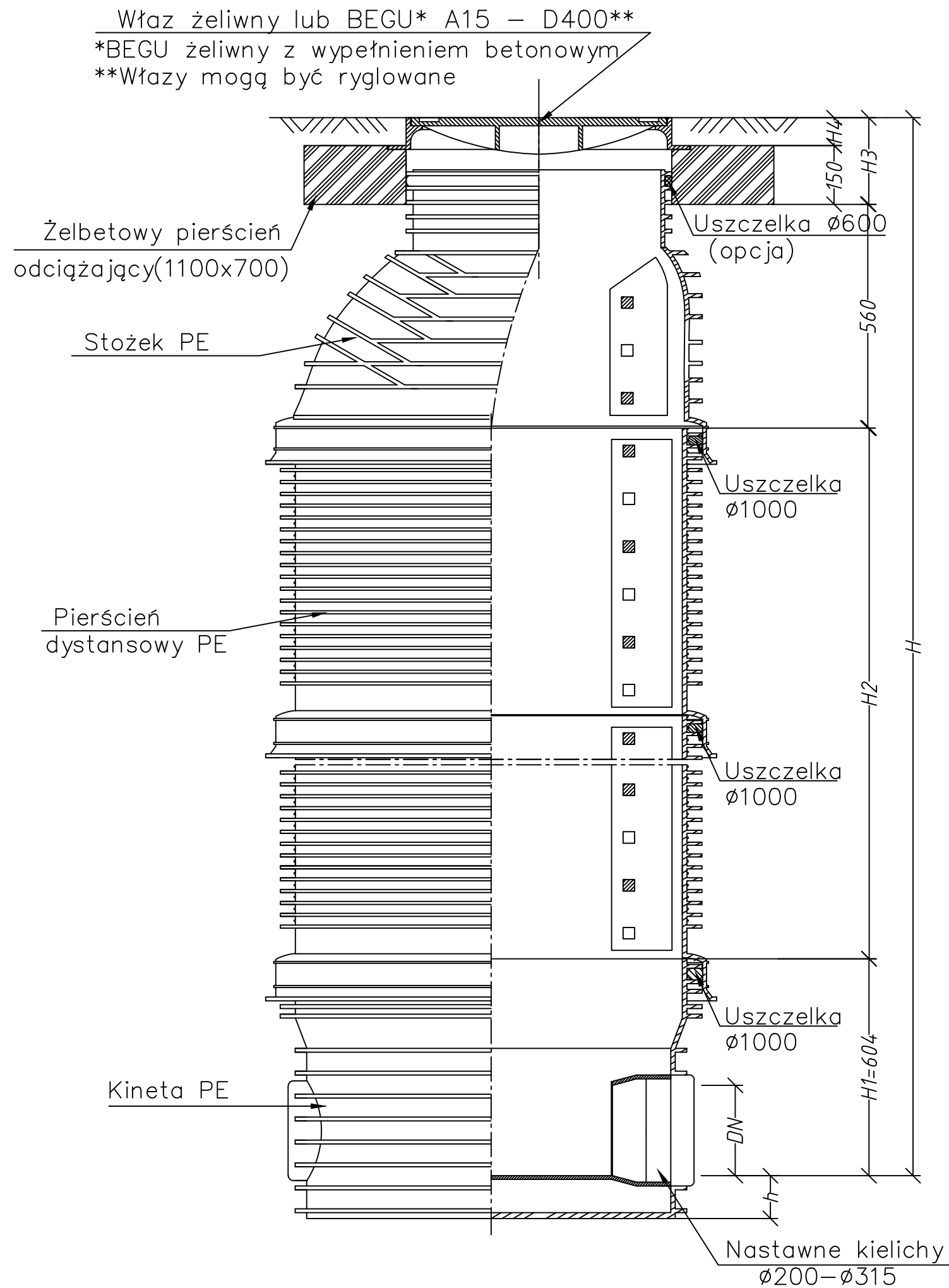
Studzienka kanalizacyjna włazowa TEGRA 1000 z nastawnymi kielichami i włazem klasy A15–D400
